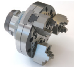
Backenmodule Gr. 145 und 215
